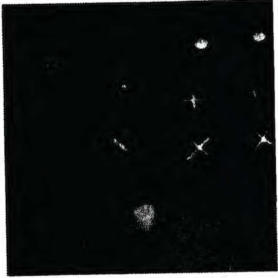
الشكل (84): ضوء يمر خلال بلورة من الكالساييت (حجر آيسلاندا) يأخذ ممرات مختلفة وفق حالة استقطابه وموضع البلورة.
